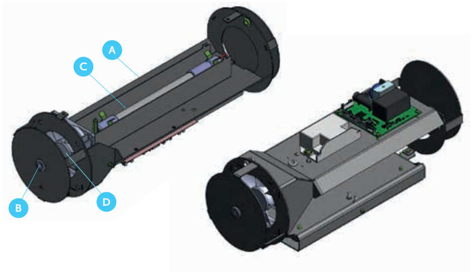
A Gehäuse · B An- / Aus-Druckschalter mit blauer Kontrollleuchte · C UV-C Spezialleuchte · D Ventilator
